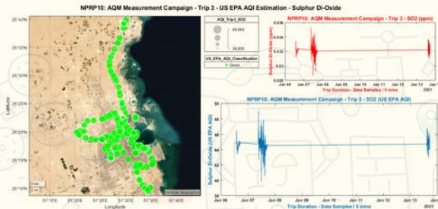
الشكل (2): جهاز رسم خرائط جودة الهواء المتنقل في الوقت الفعلي، مُركب على سيارة تويوتا كامري تقوم بدوريات في مدينة الدوحة؛ من أجل حملة رسم خرائط جودة الهواء التي قام بها الصندوق القطري لرعاية البحث العلمي.
