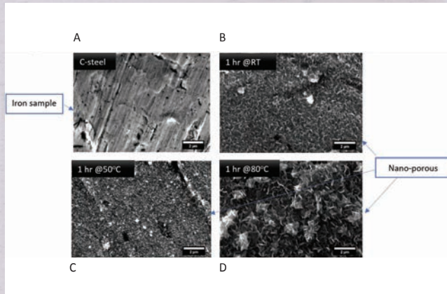
الشكل (3): تصوير المجهر الإلكتروني الماسح لـ (أ) فولاذ كربوني غير متفاعل (ب) كبريتيد الهيدروجين لمدة ساعة بدرجة حرارة الغرفة و(ج) كبريتيد الحديد لمدة ساعة بدرجة حرارة 50 مئوية (د) كبريتيد الحديد لمدة ساعة بدرجة حرارة 80 مئوية.
